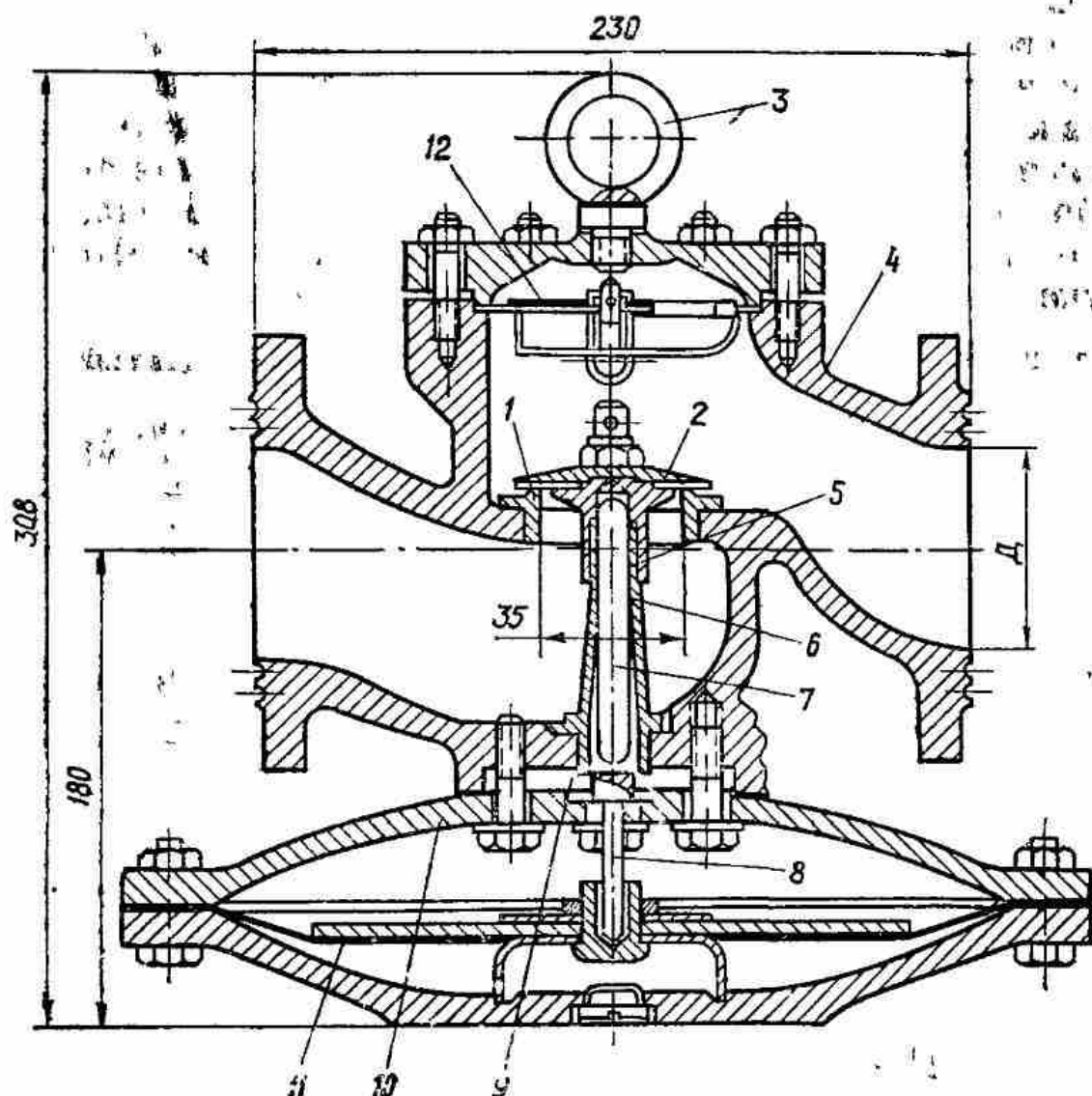
Рис. 14. Регулятор давления РДУК-2:
