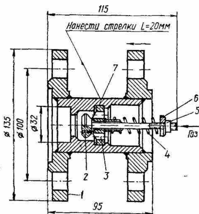
Рис 12. Скоростной клапан Ду32 автоцистерны:
