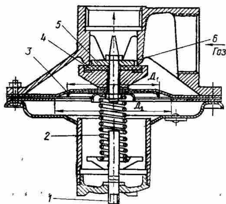
Рис. 11. Клапан ПСК.
