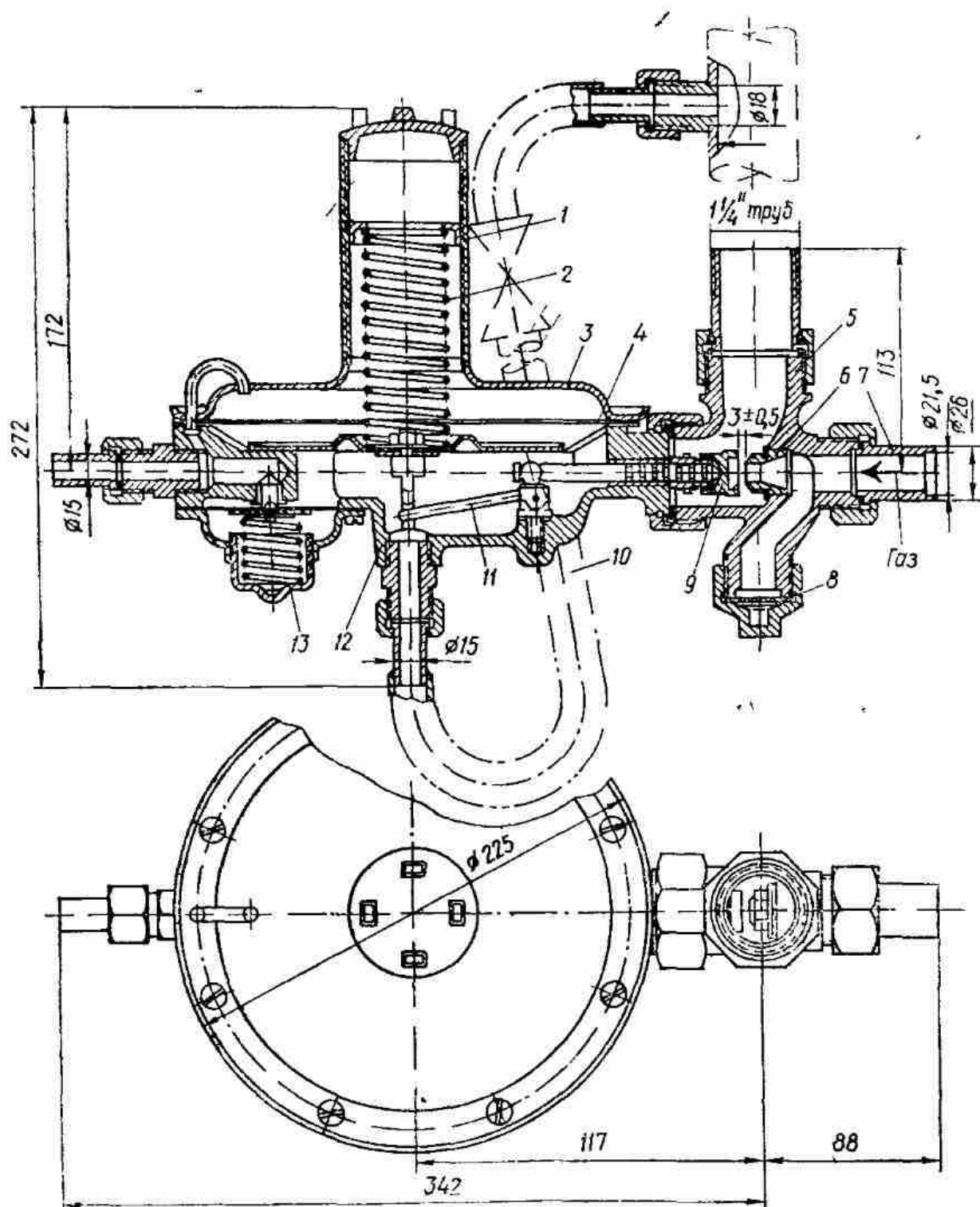
Рис. 13. Регулятор давления РД-32М:
