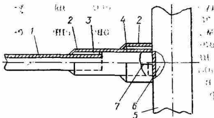
Рис. 34. Телескопическое присоединение газопровода под газом:
