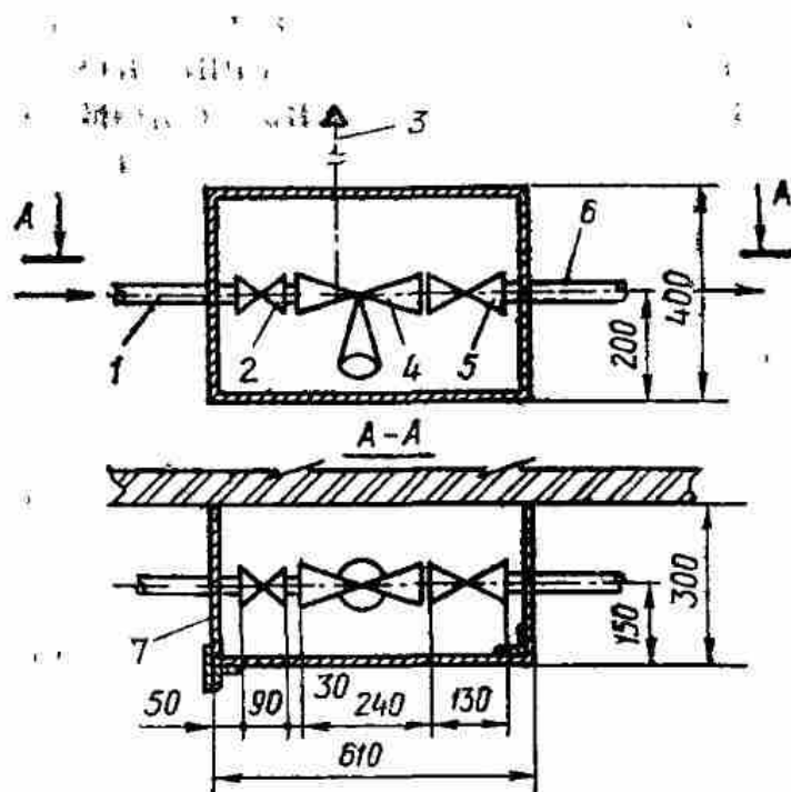
Рис. 16. Установка регулятора давления газа РДГД-20
