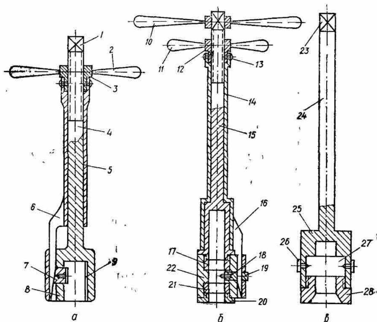
Рис. 25. Набор инструмента для ремонта сифонных стояков с конденсато-сборниками низкого давления:
