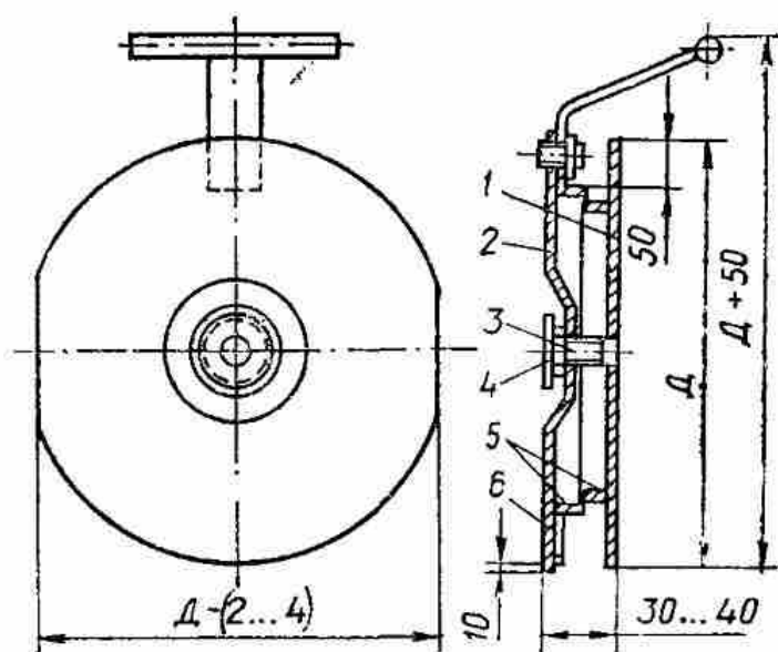
Рис. 29. Заслонка двухдисковая: 1 — диск; 2 — стальной лист; 3 — шпилька; 4 — гайка; 5 — кольцо-ограничитель; 6 — кольцо-захват.
