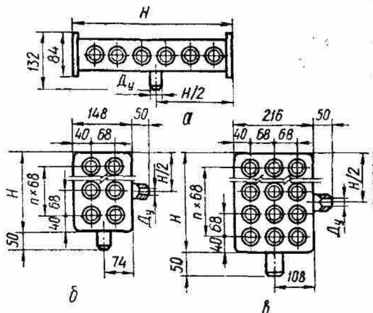
Рис. 7. Горелки БИГ-1 со смесителями однорядным (а), двухрядным (б) и трехрядным (в).
