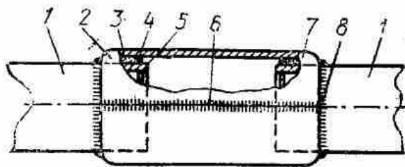
Рис. 35. Соединение газопроводов под газом при помощи разрезной подвижной муфты:
