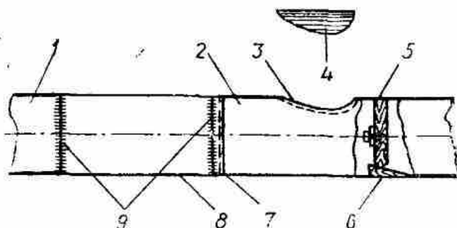
Рис. 33. Торцевое присоединение газопровода:
