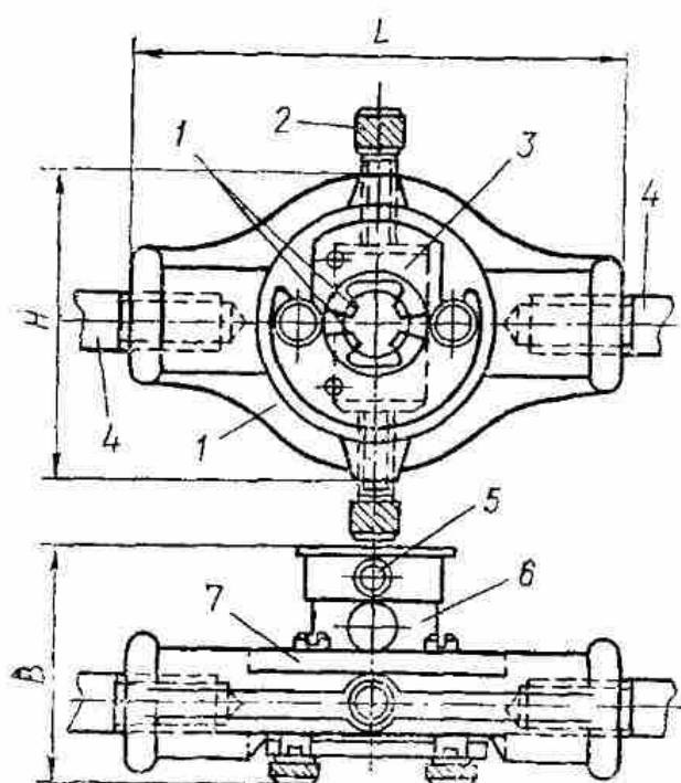
Рис. 20. Клупп конструкции Маевского для водогазопроводных труб:
