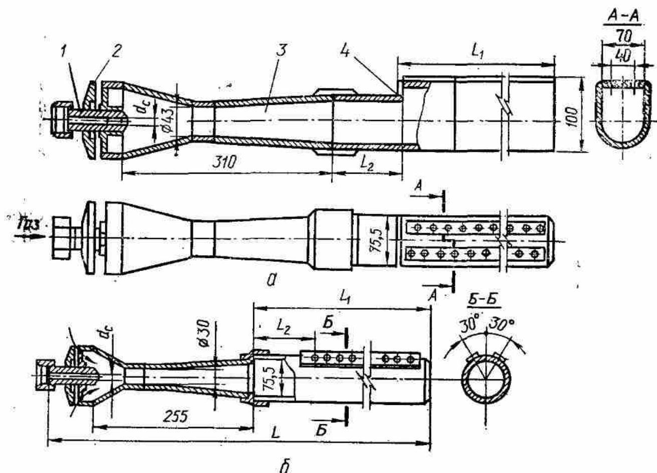
Рис. 6. Горелки ГКС-6, ГКС-8 и ГКС-10 (а) и ГКС-2,5 (б) конструкции Мосгазниипроекта:
