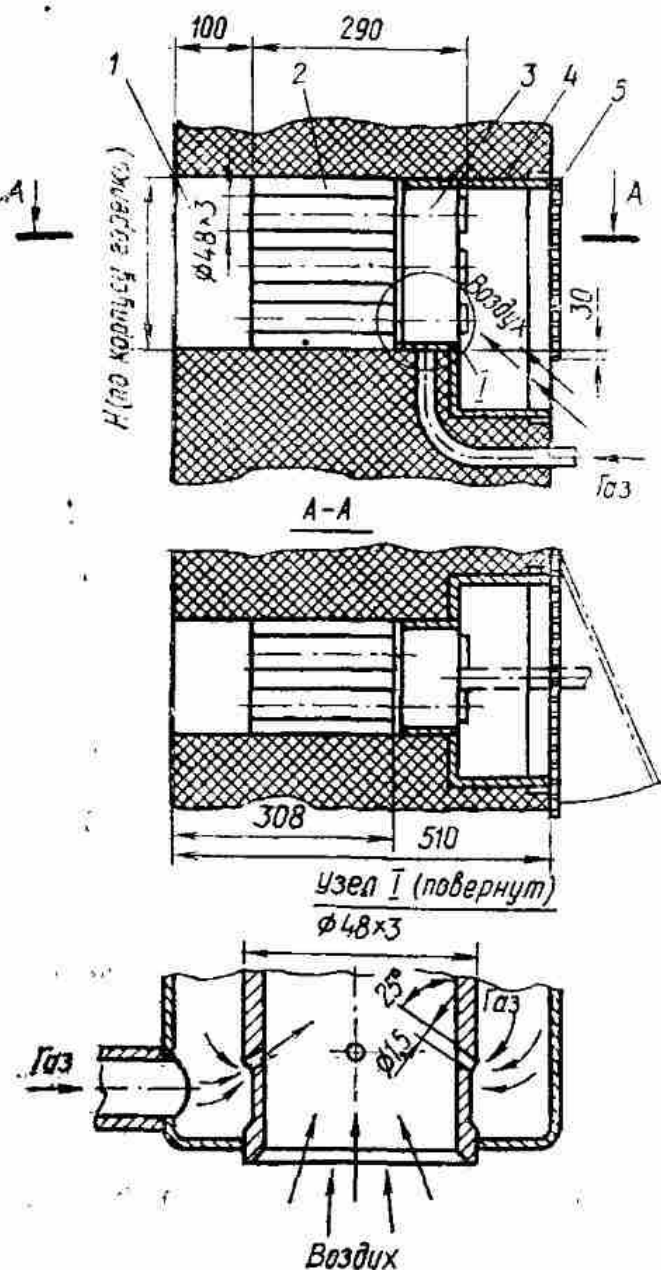
Рис. 8. Горелка среднего давления типа БИГ конструкции Промэнергогаза:
