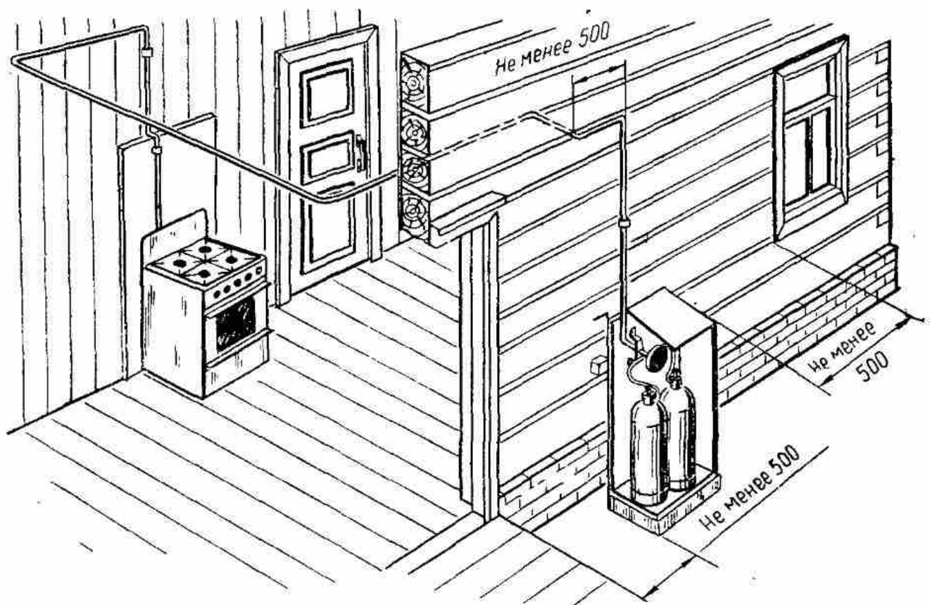
Рис. 5. Вариант размещения индивидуальной газобаллонной установки в специальном шкафу.
