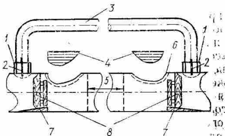
Рис. 36. Схема устройства обводной трубы для ремонта участка газопровода под газом:
