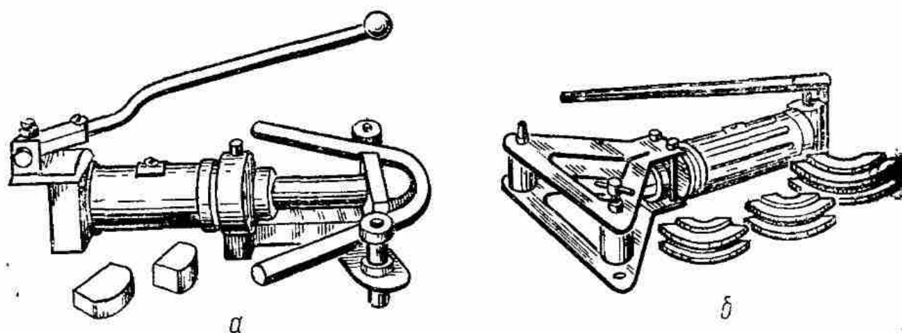
Рис. 26. Ручные гидравлические трубогибы типов ТРГ-3/4" (а) и ТРГ-2" (б)
