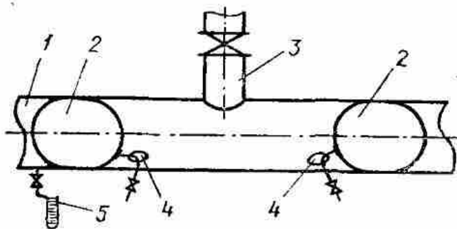
Рис. 31. Присоединение к действующему газопроводу при помощи резиновых камер:
