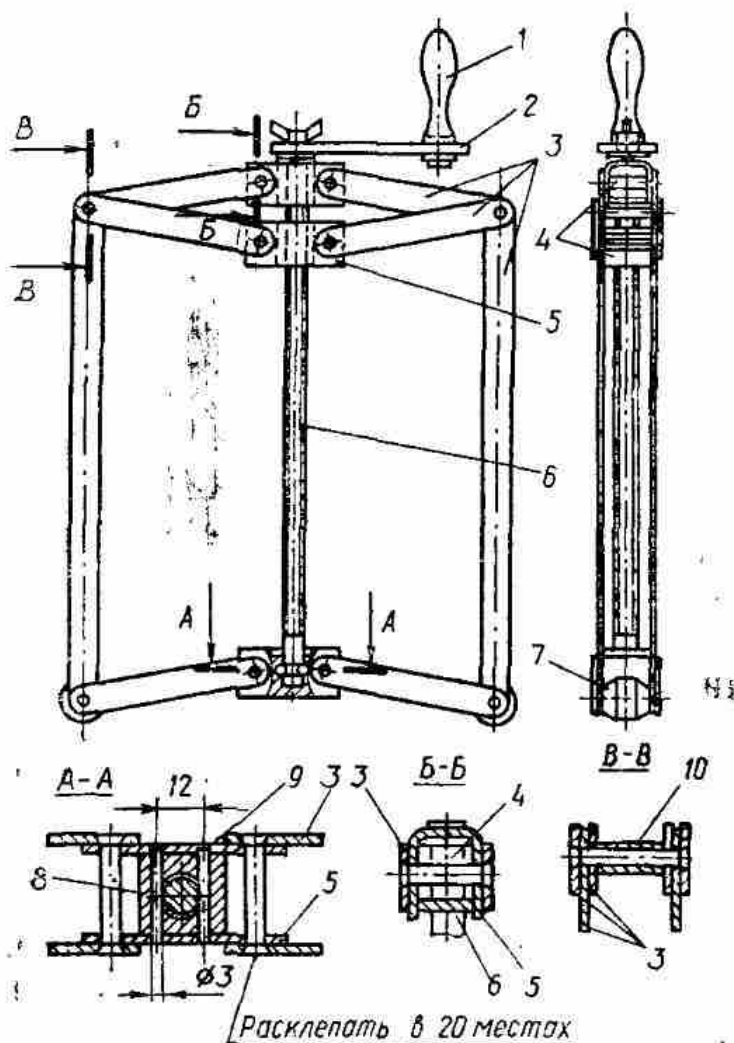
Рис. 30. Распор для заслонки:
