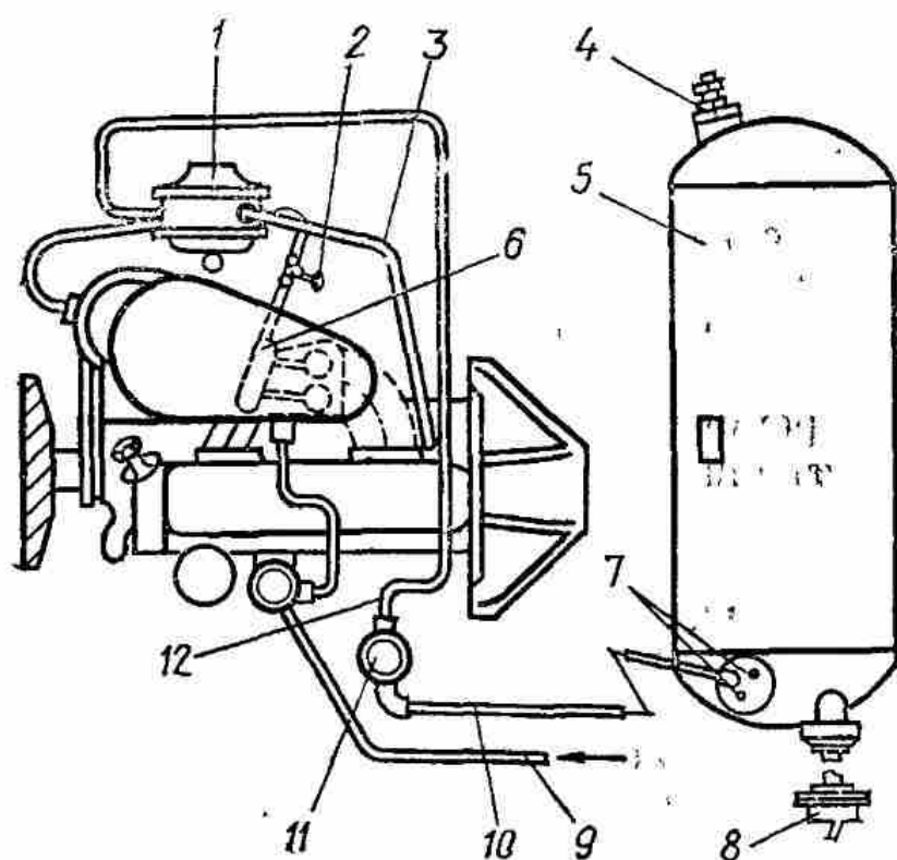
Рис. 37. Схема газобаллонной установки автомобиля ГАЗ-24-17 «Волга»:
