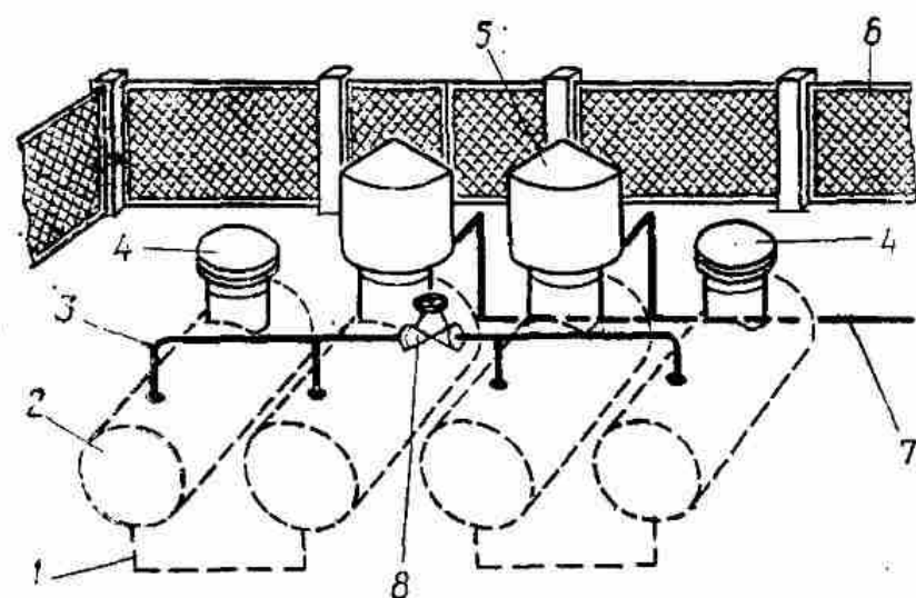
Рис. 3. Схема групповой установки из четырех резервуаров с обвязками по жидкой фазе:
