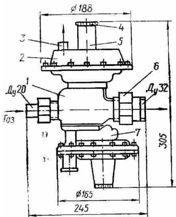
Рис. 15. Регулятор давления газа РДГД-20:
