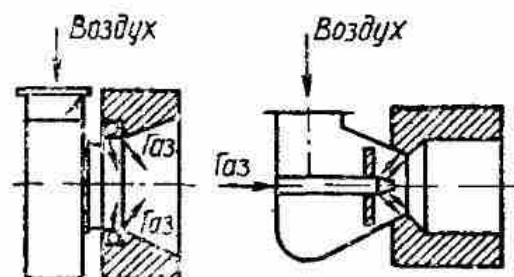
Рис. 9. Принципиальные схемы газовых горелок с принудительной подачей воздуха.
