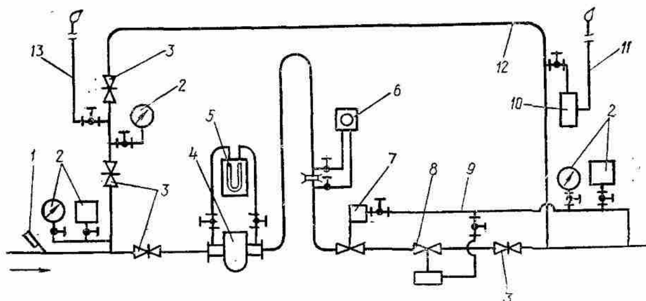
Рис. 1. Технологическая схема ГРП (ГРУ):
