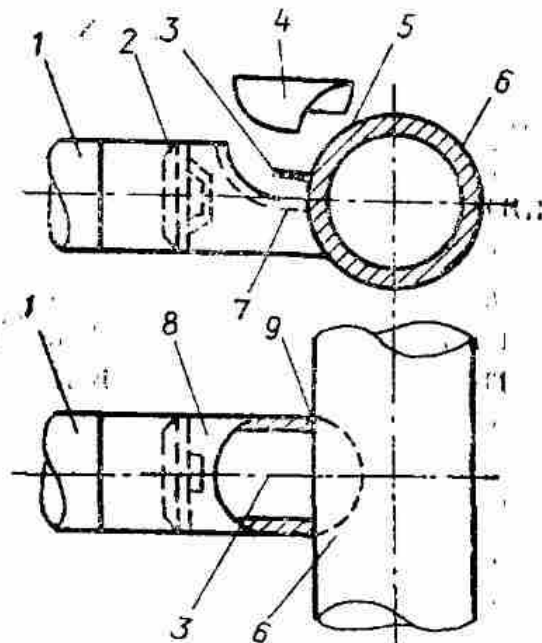
Рис. 32. Присоединение с помощью козырька (тавровое присоединение):
