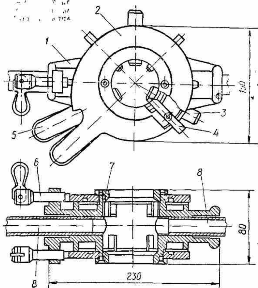
Рис. 19. Клупп газовый трубный для водогазопроводных труб:
