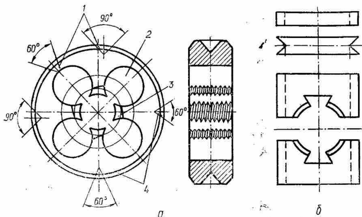
Рис. 21. Плашки круглая (а) и раздвижная (б):
