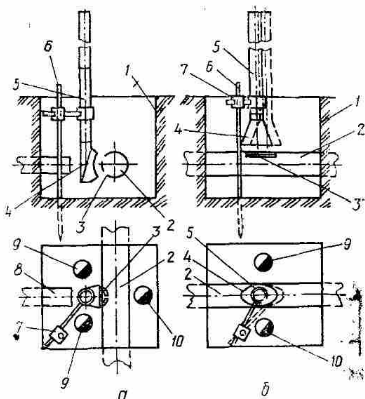
Рис. 27. Применение пламеотводной трубы при огневых работах на действующих газопроводах низкого давления:
