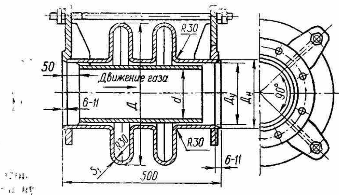
Рис. 17. Компенсатор двухлинзовый.
