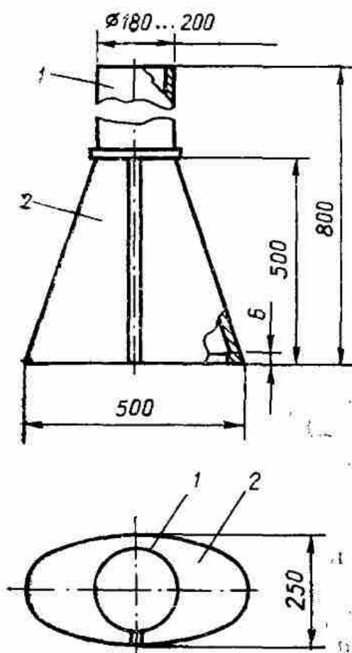
Рис. 28. Насадок пламеприемный верхний:
